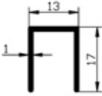
603.01 LAMBRI U SU 0,121gr/m
