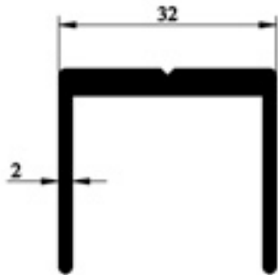
603.04 GENİŞ U BAĞLANTI 0,620gr/m
