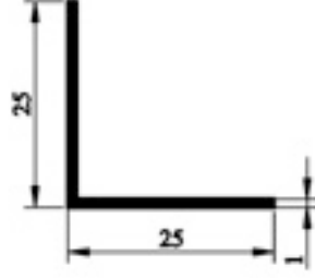
601.02 25 X 25 KÖŞEBENT 0,135gr/m
