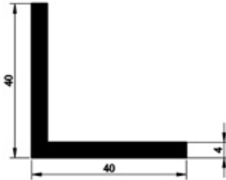
601.08 40 X 40 KÖŞEBENT 0,820gr/m
