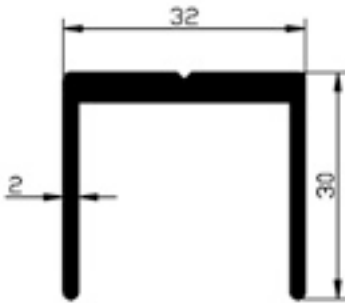
603.04 GENİŞ U BAĞLANTI 0,620gr/m
