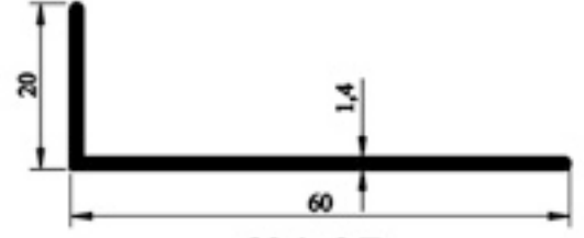
601.07 20X60 KÖŞEBENT 0,297gr/m
