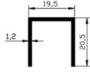
603.03 ASMA TAVAN 0,320gr/m
