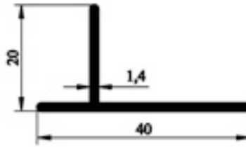
602.05 ASİMETRİK T 0,221gr/m
