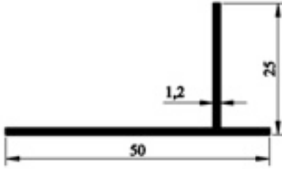
602.04 50 X 25 T 0,170gr/m
