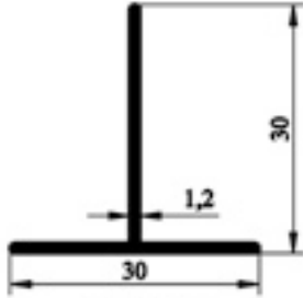
602.01 30 X 30 T PROFİLİ 0,180gr/m
