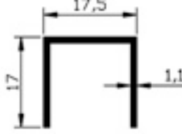
603.02 DAR PANJUR U PROFİLİ 0,175gr/m
