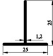
602.02 25 X 25 T PROFİLİ 0,145gr/m
