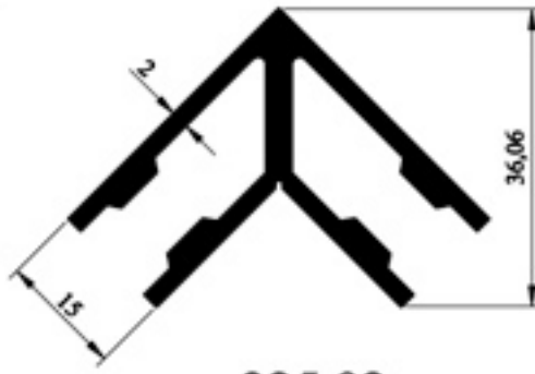
325.02 DAR ÇAVUŞ KÖŞE 0,860gr/m
