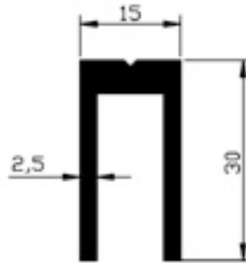
603.05 DAR U BAĞLANTI 0,540gr/m
