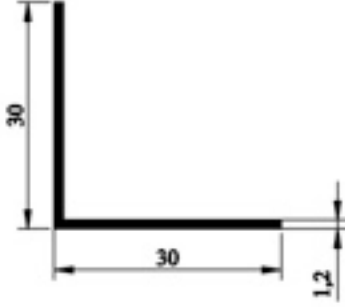
601.01 30 X 30 KÖŞEBENT 0,175gr/m
