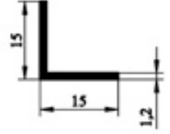
601.04 15 X 15 KÖŞEBENT 0,095gr/m
