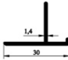
602.07 ASİMETRİK T 0,189gr/m
