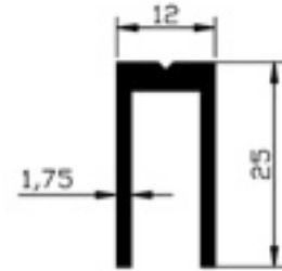
603.06 SÜRME U BAĞLANTI 0,310gr/m
