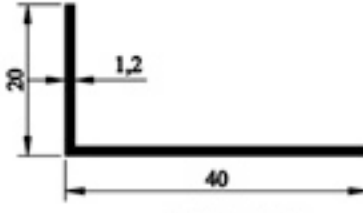
601.06 40 X 20 KÖŞEBENT 0,175gr/m
