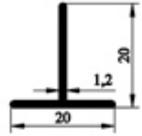
602.03 20 X 20 T PROFİLİ 0,125gr/m
