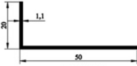
601.05 50 X 20 KÖŞEBENT 0,204gr/m
