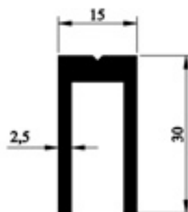
603.05 DAR U BAĞLANTI 0,540gr/m
