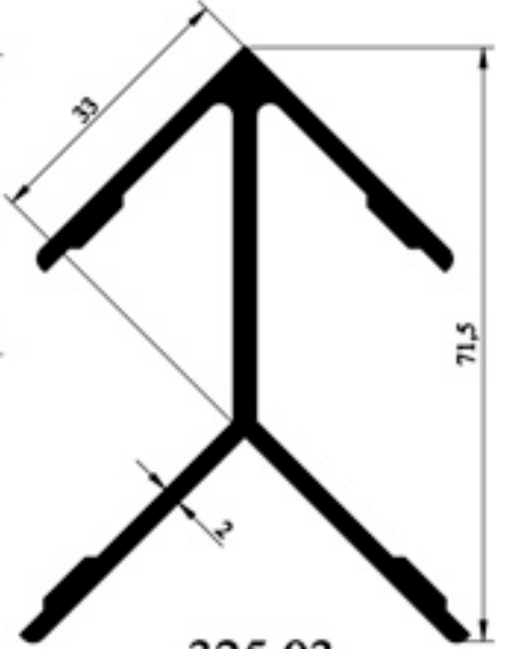
325.03 GENİŞ ÇAVUŞ KÖŞE 1.160gr/m
