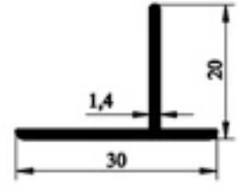
602.06 ASİMETRİK T 0,181gr/m
