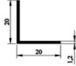
601.03 20 X 20 KÖŞEBENT 0,120gr/m
