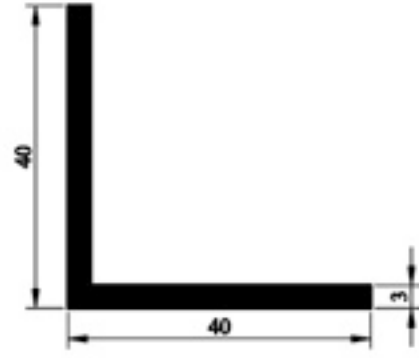
601.09 40 X 40 KÖŞEBENT 0,620gr/m
