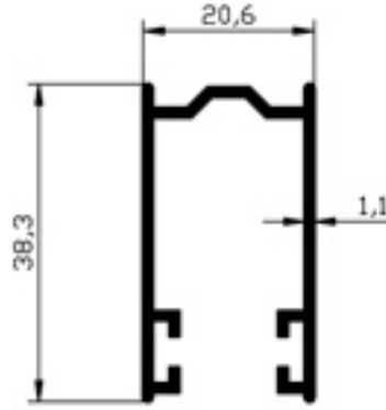
108.11 STOR U PROFİLİ 0.348gt/m
