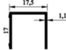
603.02 DAR PANJUR U PROFİLİ 0,175gr/m
