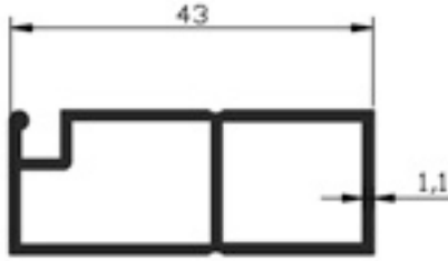
108.04 KAPI SİNEKLİK 0,404gr/m
