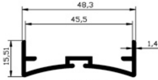
207.01 ÇARPMA KAPI ADAPTÖRÜ 0,360 gr/m
