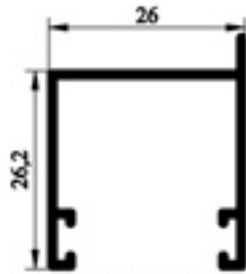
107.48 FİTİLLİ U PROFİLİ 0,256 gr/m
