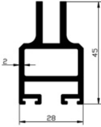
104.01 KANAT PROFİLİ 0.890gr/m
