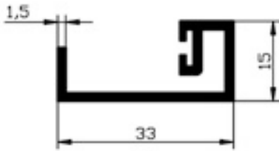
104.06 BALKON CAM KENET 0,313gr/m
