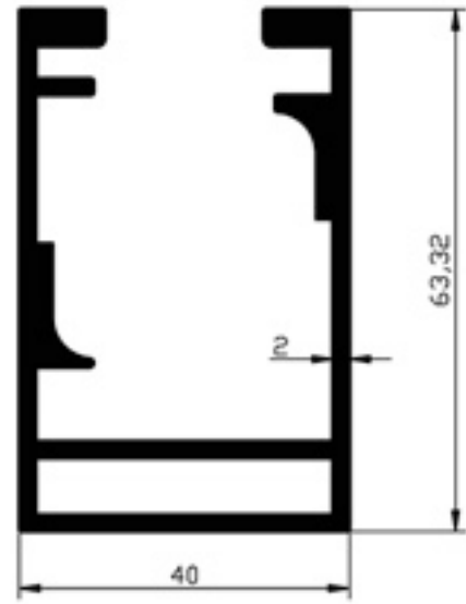
104.02 KASA PROFİLİ 1.549gr/m
