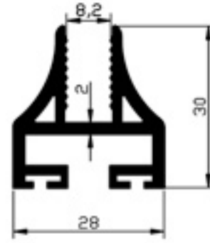
104.05 BALKON CAM YATAĞI 0,647gr/m
