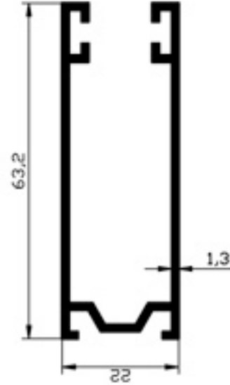
108.17 0.625gr/m STOR U PROFİLİ
