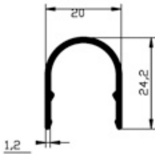
207.05 20'LİK GRİYAJ 0,200 gr/m
