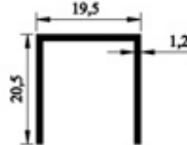
603.03 ASMA TAVAN 0,320gr/m
