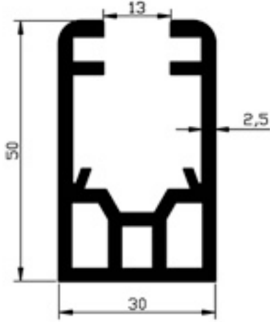
104.04 BALKON CAMLAMA KASA 1.300gr/m
