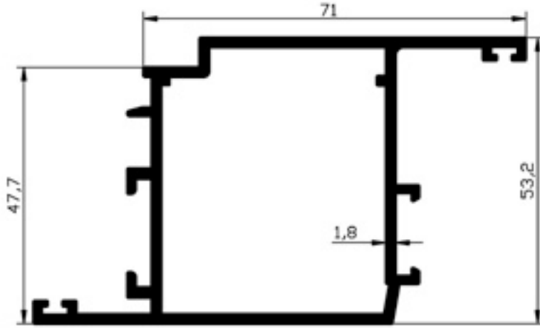
301.01 KANAT PROFİLİ 1.356gr/m
