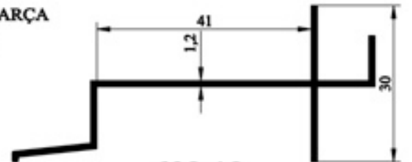
602.12 DENİZLİKLİ T PROFİLİ 0,390gr/m
