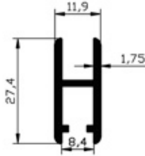
201.19 0.297gr/m H PROFİLİ
