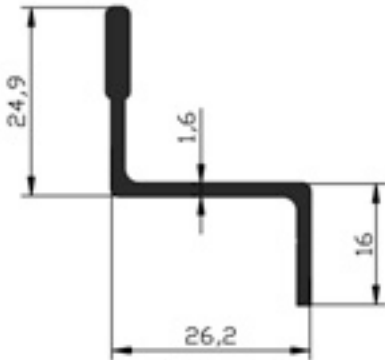
108.07 S. SİNEKLİK RAY 0.330 gr/m
