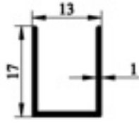
603.01 LAMBRI U SU 0,121gr/m
