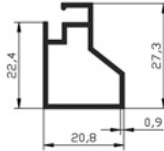
108.03 SİNEKLİK 0,233gr/m
