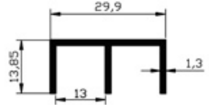
201.20 0.237gr/m B PROFİLİ
