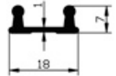
201.23 0.126gr/m RAY PROFİLİ
