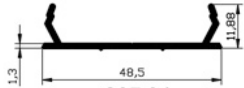
207.04 50'LİK GRİYAJ ALTI 0,250 gr/m
