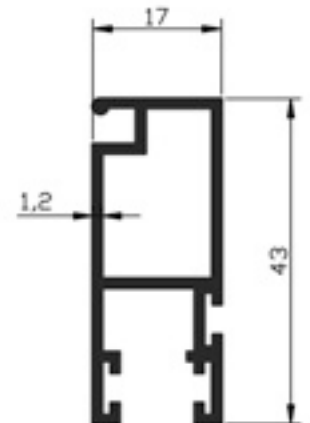
108.09 SÜRME SİNEKLİK 0.460 gr/m
