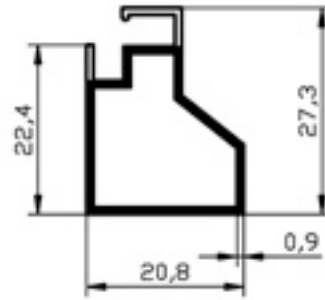
108.03 SİNEKLİK 0,233gr/m
