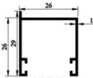
107.01 FİTİLLİ U PROFİLİ 0,254gr/m
