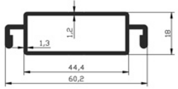
108.02 ÇİFT KULAKLI SİNEKLİK 0,563gr/m
