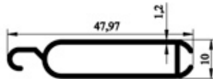
107.02 FİTİLLİ ALT PARÇA 0,350gr/m
