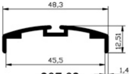
207.02 ÇARPMA KAPI ADAPTÖRÜ 0,330 gr/m
