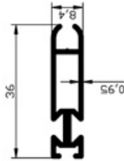
108.16 0.275gr/m STOR ALT PARÇA
