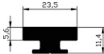
104.03 BAĞLANTI 0.513gr/m
